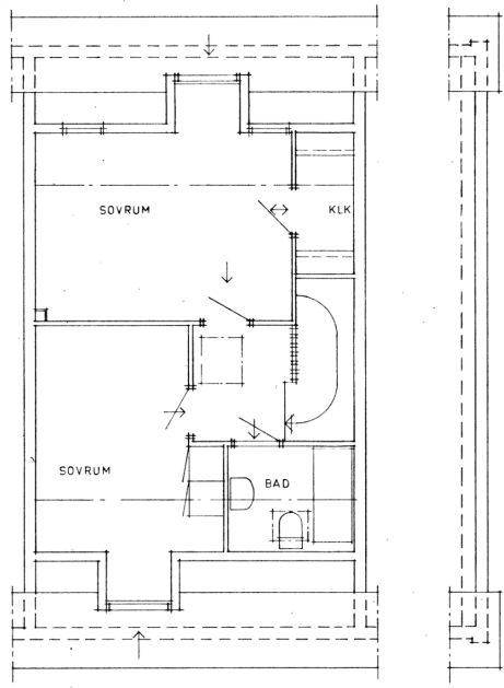
VINDSPLAN
