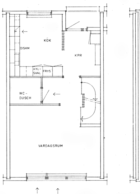
ÖVERPLAN (ENTREPLAN)
