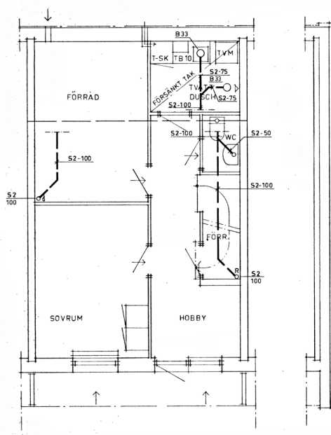
SUTERRÄNGPLAN
