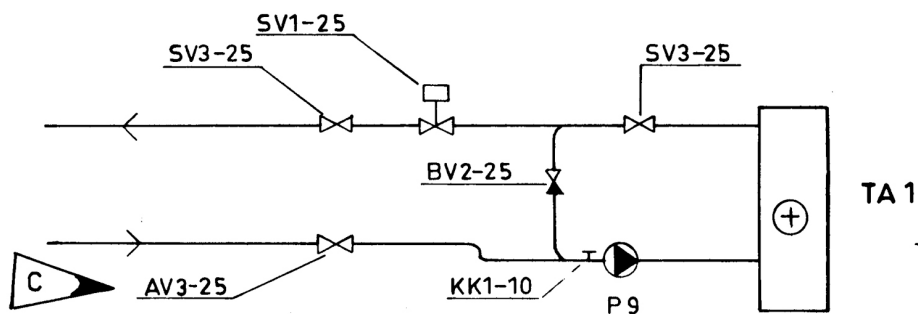
PRINCIP KOPPLINGSSCHEMA
